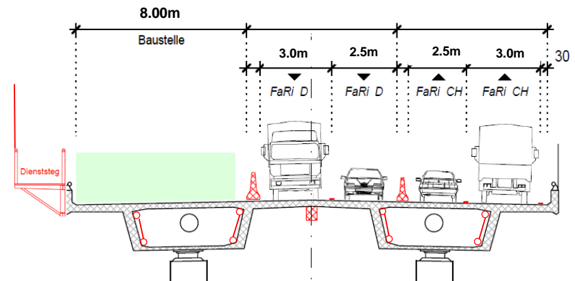
Bauphase 3
