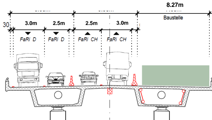
Bauphase 2
